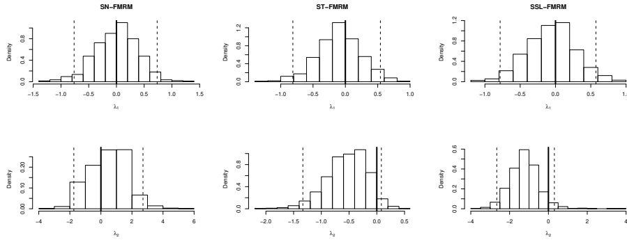
Figure 3: Skewness parameters posterior samples.
